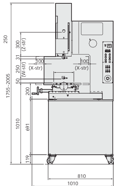
Elnézet
