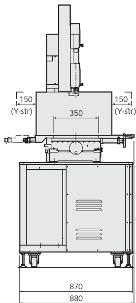
Oldalnézet
